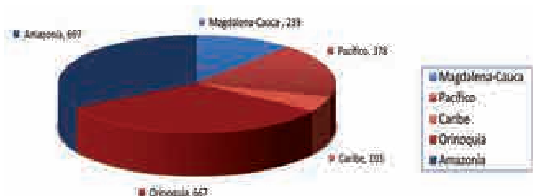
Figura 3.1 Volumen de agua en áreas hidrográficas representativas, Km3.
