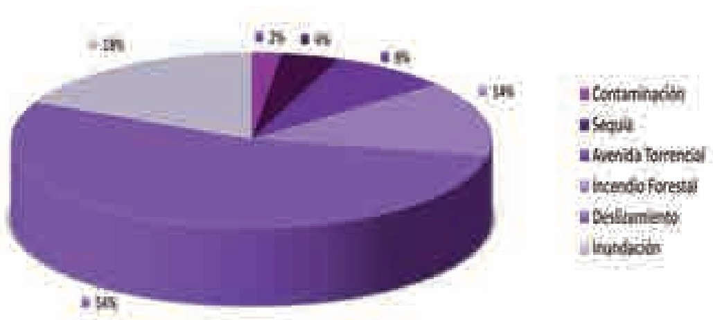
Figura 3.17 Registro de desastres relacionados con el agua. 1987 – 2007.
