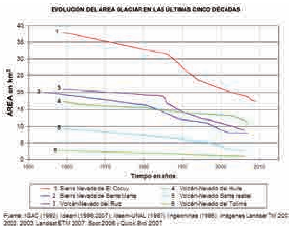
Figura 3.6 Evolución del área glaciara de los seis nevados existentes en Colombia
