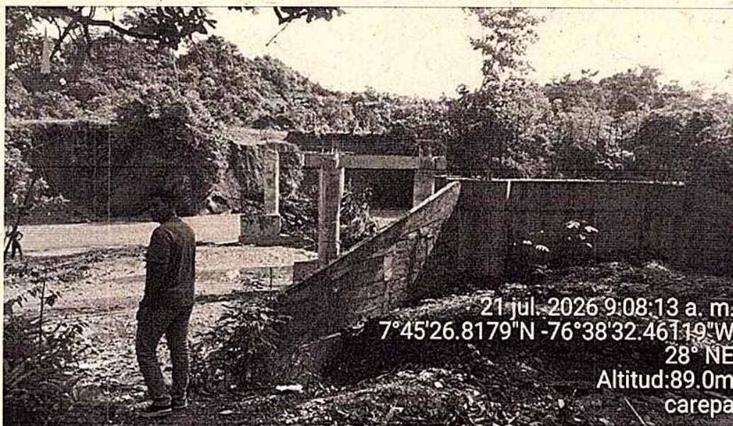
Foto 3: Estribo de la margen izquierda y dos estructuras con dos pilotes construidos sobre el cauce del río Carepa.
