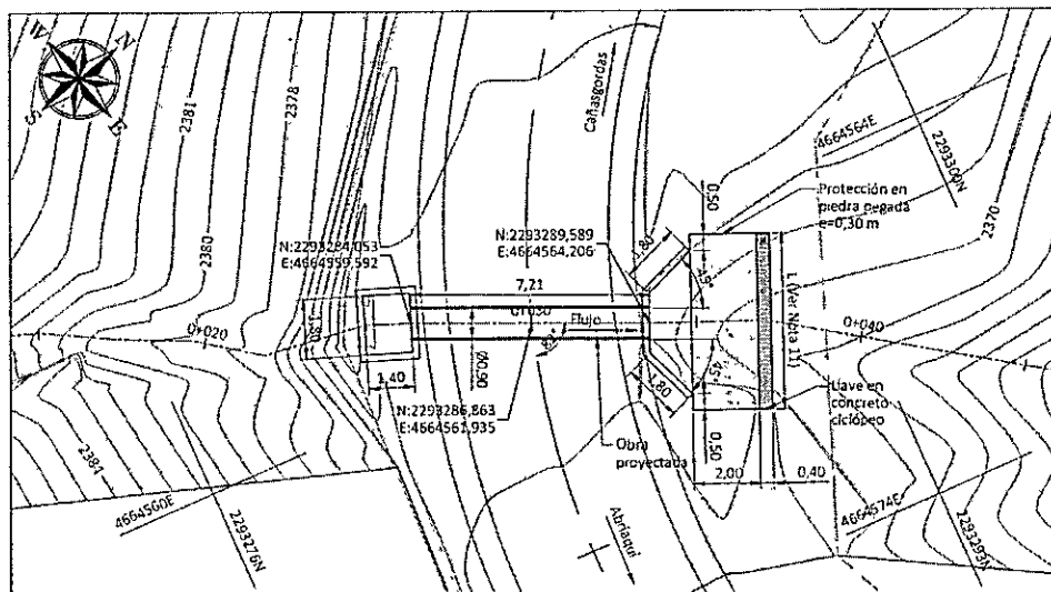
ID 43 ALCANTARILLA Ø0,90 m K19+353 INTERVENCIÓN: PROPUESTA PLANTA ESCALA 1:150
