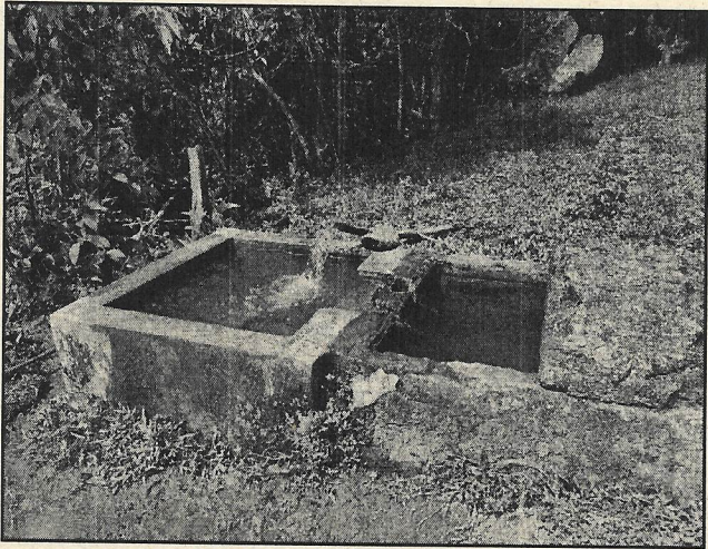
Imagen 3. Desarenador
